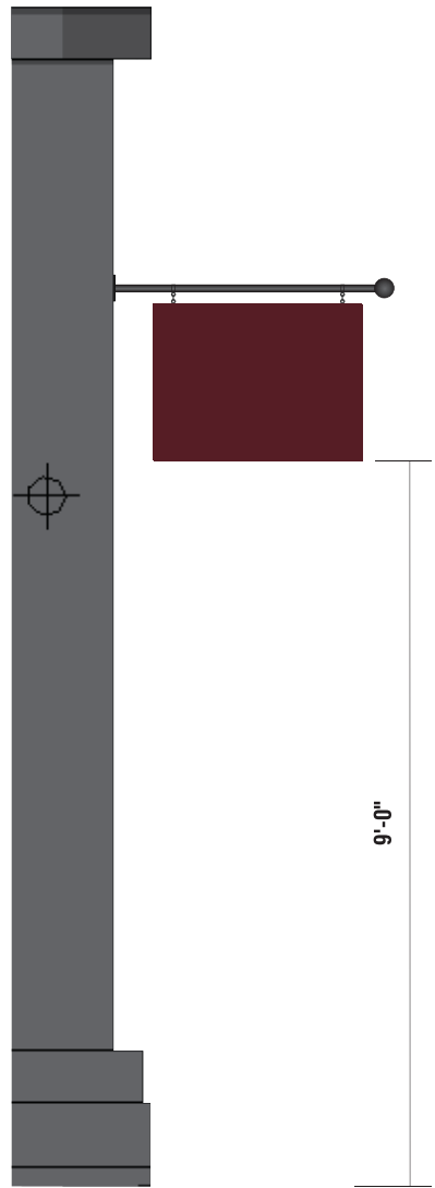
2 COLUMN SIDE VIEW SCALE: 3/8" = 1'-0"
